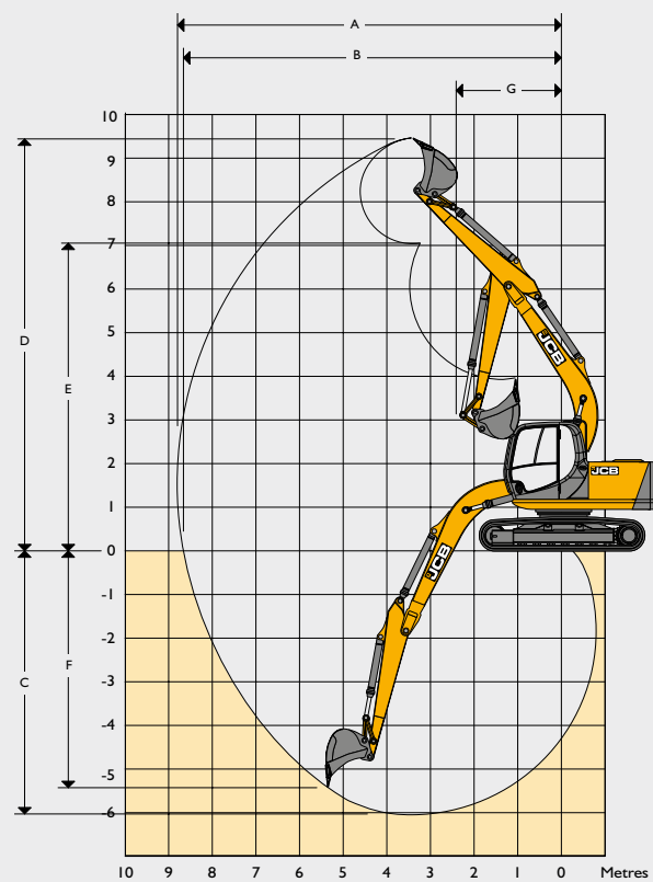
JSI 30/145 MONOBOOM
