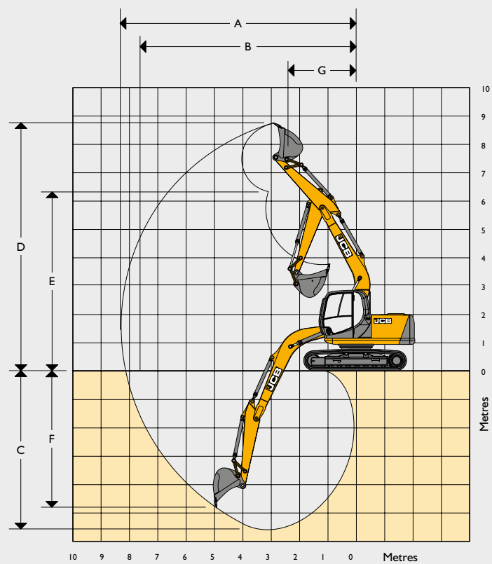
JSI 115 MONOBOOM
