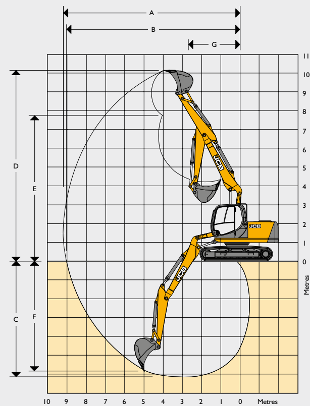
JSI 30/145 TAB
